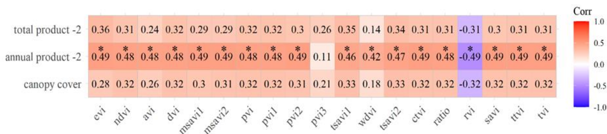
شکل ۶- بررسی ارتباط شاخص‌های گیاهی تصویر Landsat-8 تولید کل
