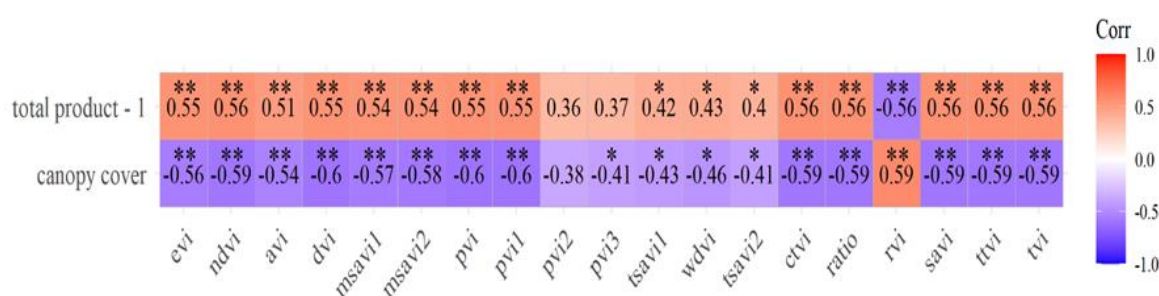
شکل ۳- بررسی ارتباط شاخص‌های گیاهی تصویر Landsat-8 با تولید کل Product 1 و Canopy cover 1: به ترتیب درصد پوشش گیاهی و تولید دوره اول نمونه‌برداری (فروردین)
