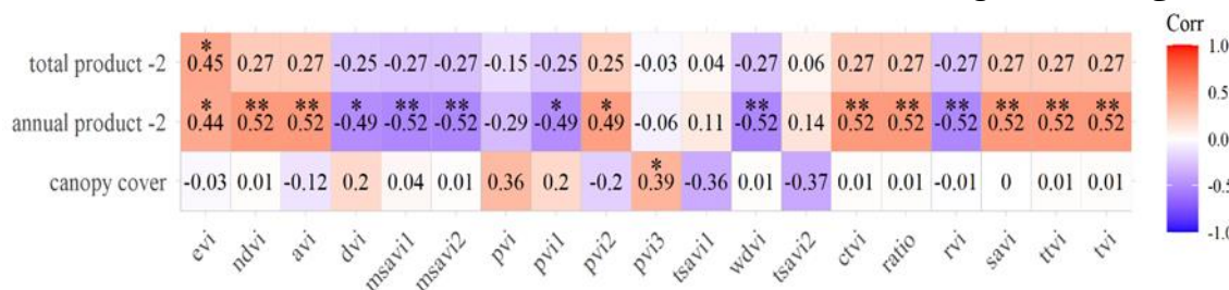
شکل ۱۰- بررسی ارتباط شاخص‌های گیاهی تصویر Landsat-8 با تولید کل
