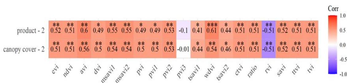
شکل ۵- بررسی ارتباط شاخص‌های گیاهی تصویر Landsat-8 با شکل رویشی PG
