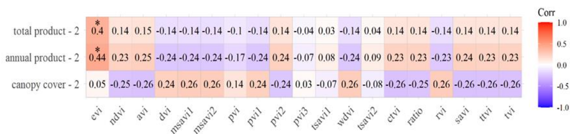
شکل ۹- بررسی ارتباط شاخص‌های گیاهی تصویر Landsat-8 با شکل روشی SH
