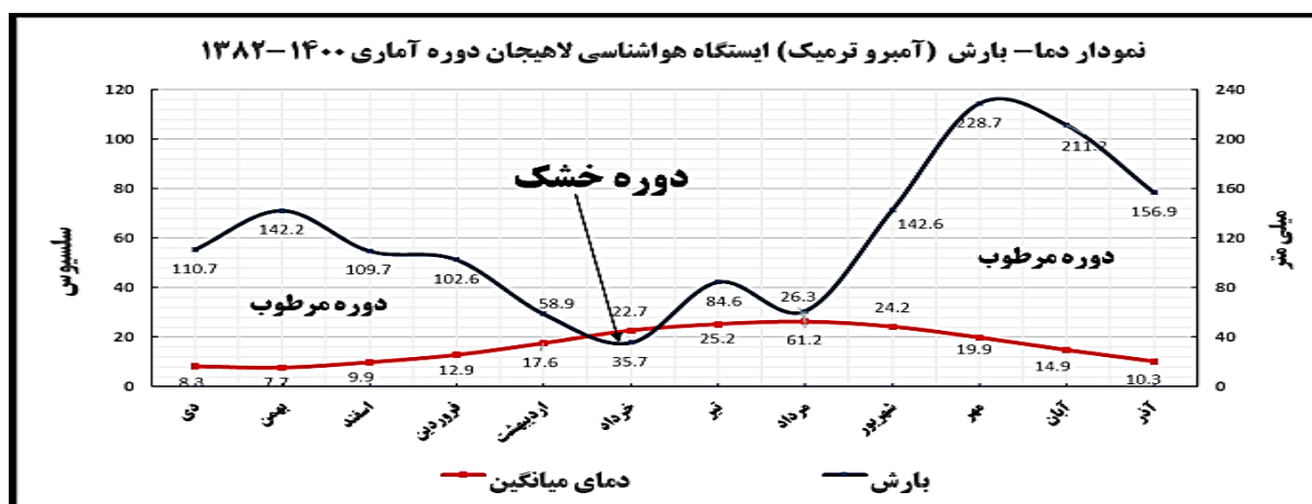
شكل ۲- نمودار دما - بارش (منحنى آمبروترميك) ايستگاه سينوپتيك تكميلى شهرستان لاهيجان (۱۴۰۰-۱۳۸۲) (گروه توسعه هواشناسى کاربردى، ۱۴۰۲)
