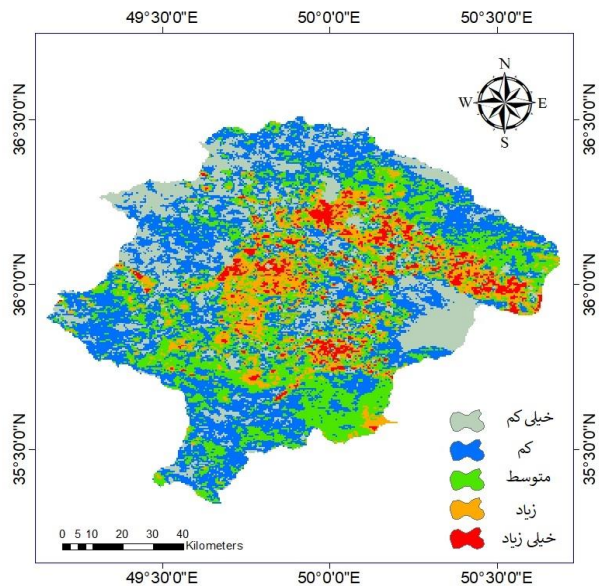
شکل ۱۲- حساسیت NPP به انحراف معیار دما (ورود تمام پارامترها به معادله)
