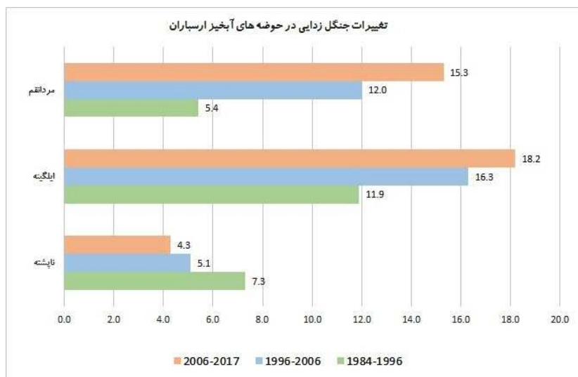
شکل ۴- نمودار تغییرات میزان کاهش جنگل در حوضه‌های آبخیز ارسباران طی سه دوره زمانی
