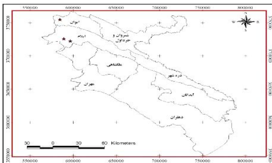
شکل ۱- نقشه پراکنش گونه زوفایی در استان ایلام
