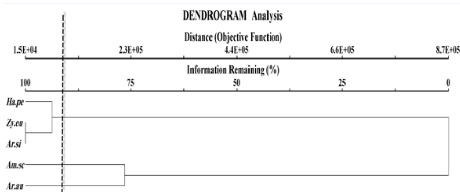
شکل ۳- دندروگرام آنالیز خوشه‌ای با استفاده از روش مجذور فاصله اقلیدسی بر پوشش گیاهی مراتع غرب تفتان
