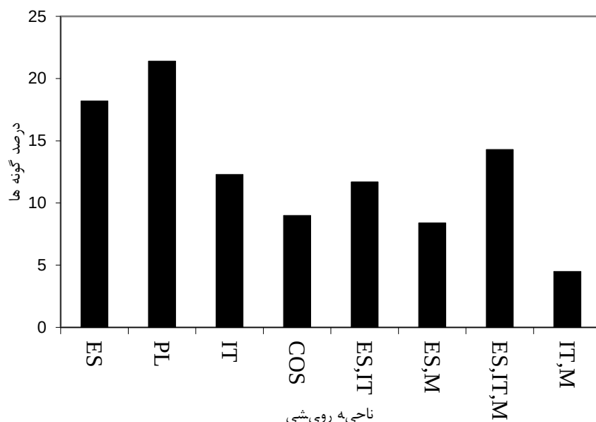
شکل ۴- پراکندگی جغرافیایی گونه‌های گیاهی اراضی مرتعی حوضه توتکابن، ES = اروپا- سبیری، IT = ایرانی- تورانی، M = مدیترانه‌ای، PL = چند ناحیه‌ای، Cosm = جهان وطن
