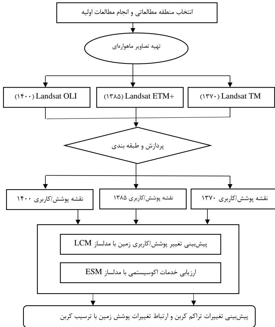
شكل ۲- مراحل ارزيابي و تحليل كاريبي/پوشش زمين
