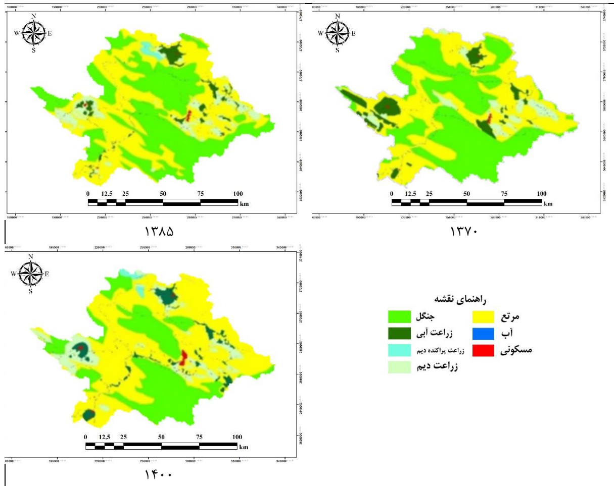
شکل ۲- تغییرات پوشش زمین در سه دوره زمانی ۱۳۷۰، ۱۳۸۵ و ۱۴۰۰
