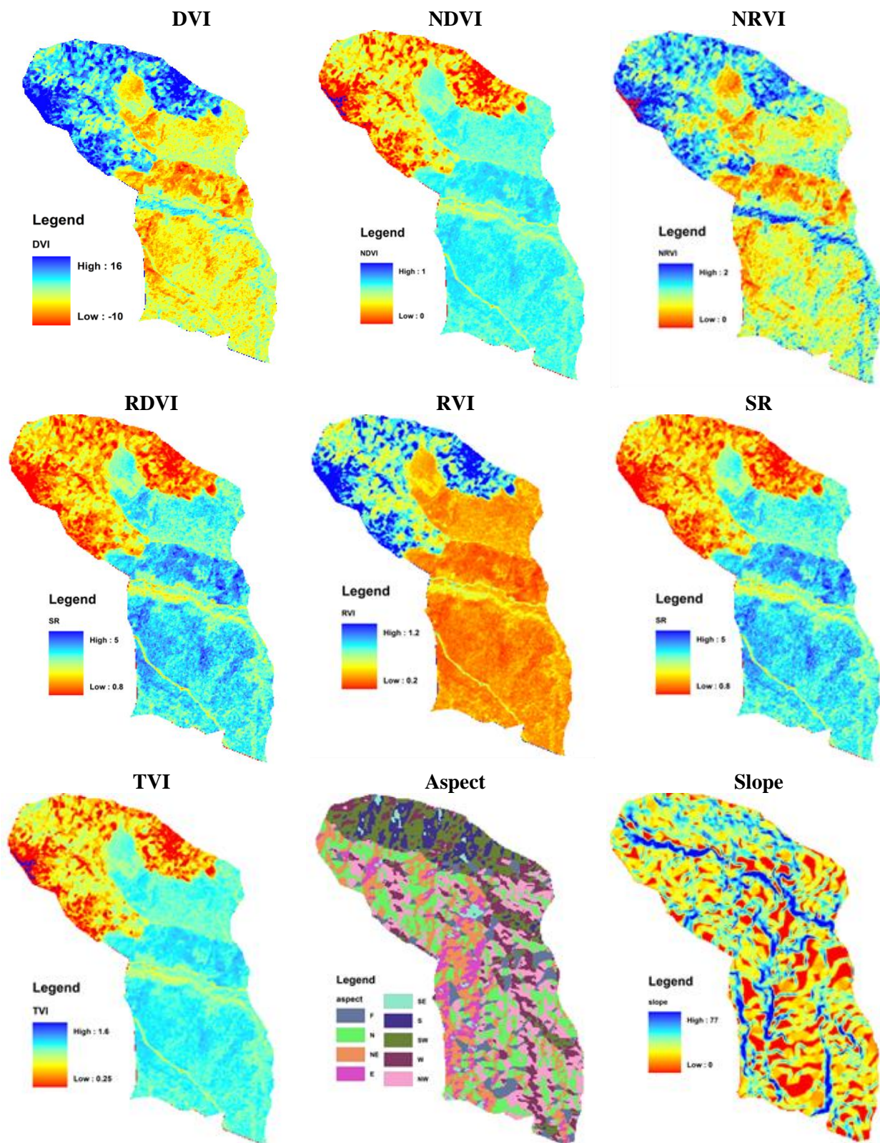
شکل ۳- نقشه‌های شاخص‌های پوشش گیاهی و فیزیوگرافی
