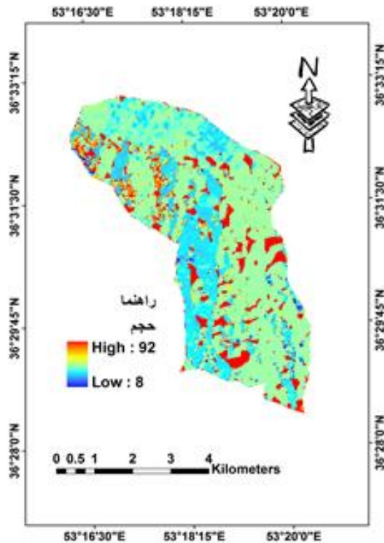
شکل ۶- نقشه حجم توده سرپا (مترکعب درهکنار) جنگل آموزشی و پژوهشی دارابکلا با استفاده از رگرسیون چندمتغیره
