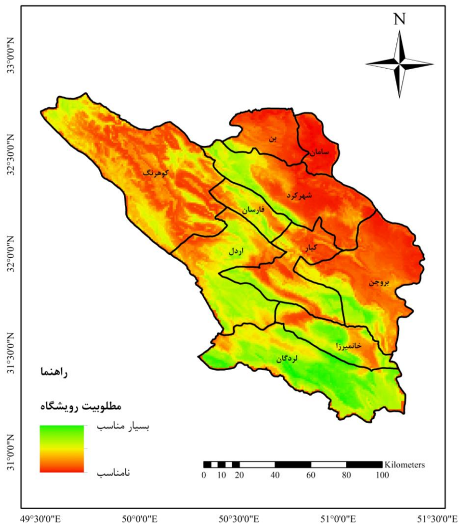
شکل ۲- مطلوبیت رویشگاه گونه جاشیر ( P. ferulacea ) بر اساس رویکرد اجماعی حاصل از پنج مدل پراکنندگی گونه‌ای
