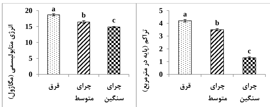
شکل ۵- نتایج مقایسه میانگین اثر شدت چرا بر مقدار انرژی متابولیکی و تراکم گونه B. tomentellus
