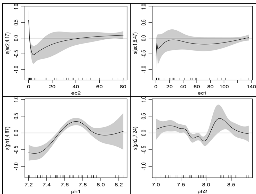
شکل ۳- رابطه برخی از متغیرهای محیطی معنی دار در مدل جمعی تعمیم یافته با حضور گونه A.sieberi
