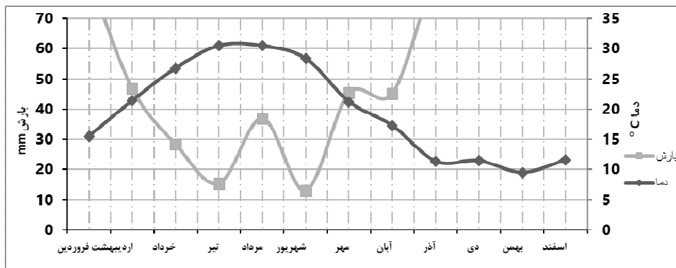
شکل ۲- منحنی آمپروترمیک ایستگاه هواشناسی مینودشت در طی دوره آماری ۱۳۹۳-۹۷
