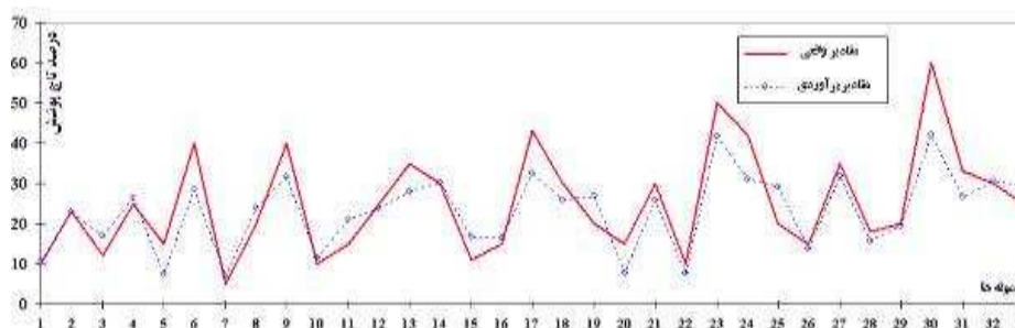
شکل ۶- ارزیابی کارایی شبکه عصبی در شبیه‌سازی میزان تاج پوشش در مرحله تست یا آزمون از طریق مقایسه مقادیر واقعی و مقادیر شبیه‌سازی شده
