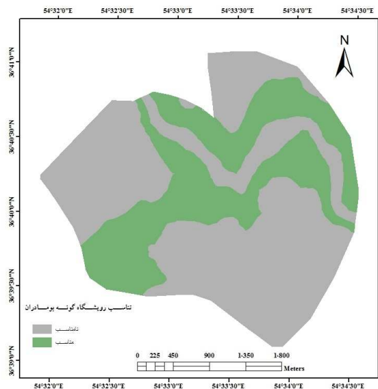
شکل ۱۶- نقشه تناسب (پتانسیل) رویشگاه گونه A. millefolium با روش رگرسیون لجستیک
