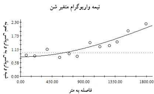
شکل ۶- نیم‌تغییرنمای درصد شن به وسیله مدل گاسن
