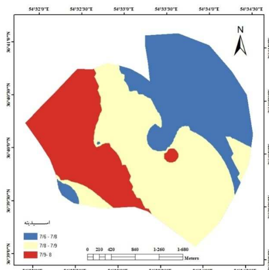
شکل ۱۲- نقشه توزیع اسیدپایه با استفاده از روش کریجینگ
